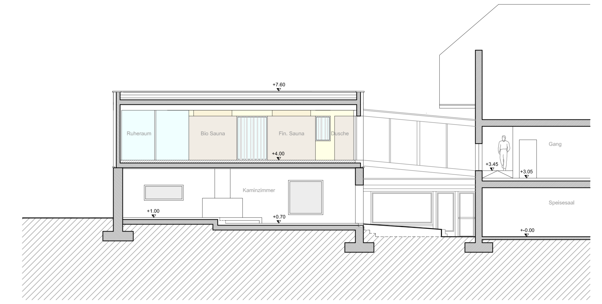
Schnitt A - A
