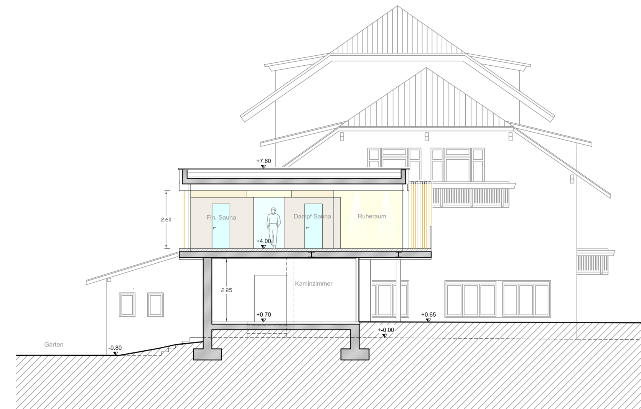
Schnitt B - B
